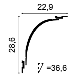
C990 + 2x P9900
