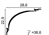
C990 + 2x P9900 90°
