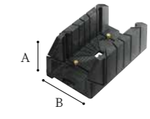
FB13 A: 12,5 cm | B: 15,5 cm
